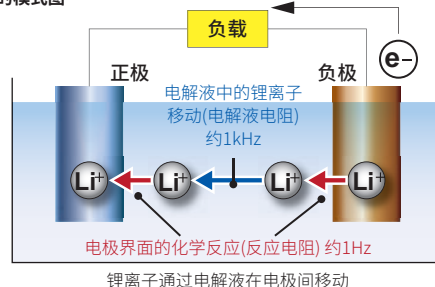
锂离子通过电解液在电极间移动
