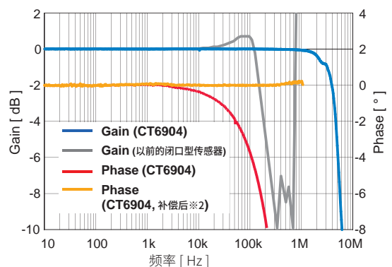
AC/DC电流传感器CT6904频率特性(代表值)
