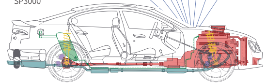
AC 非接触电压探头 SP3000
