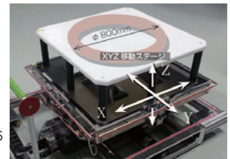
可自动控制最大直径 800mm 的大型传输线圈
